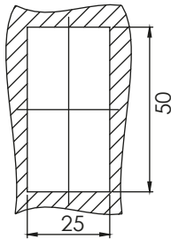
Монтажен отвор
