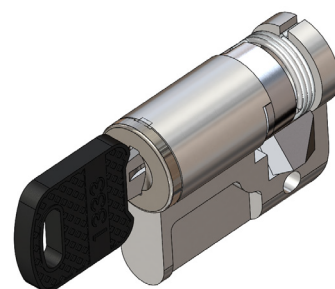
Еднаква секретност 1333 и различна секретност / в комплект с 2 ключа
