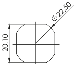
Монтажен отвор
