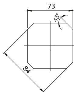
Монтажен отвор
