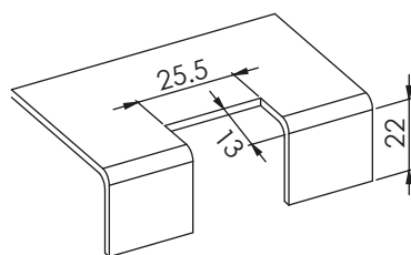
Монтажен отвор
